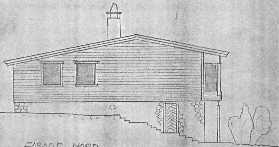
FASADE NORD.
